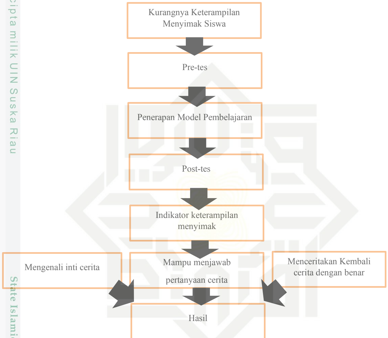
Gambar 2. 1 Kerangka Berpikir
