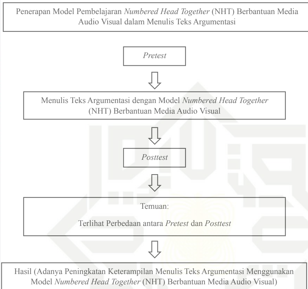
Gambar 1.1 Kerangka Berpikir
