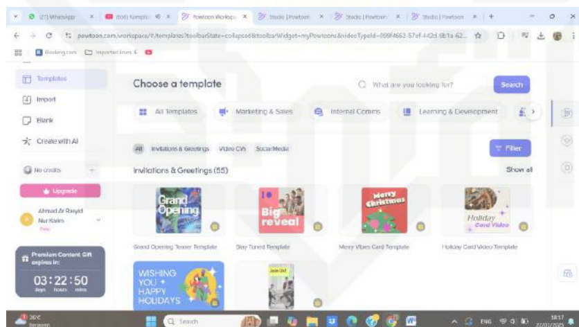
Gambar II. 9 Menu Template
