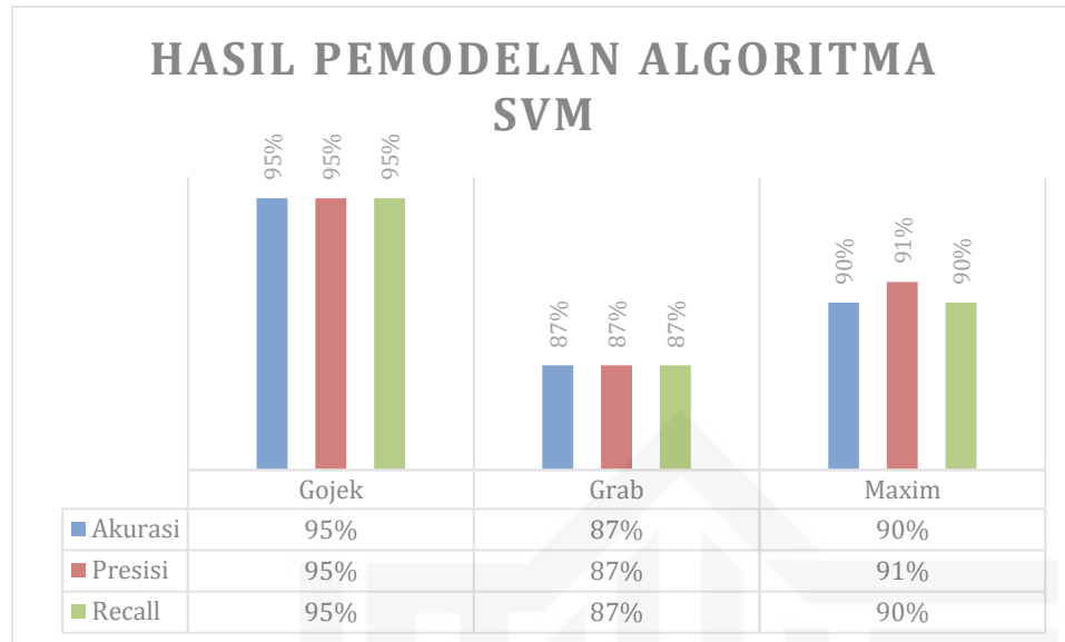
Gambar 2. Hasil Evaluasi Model SVM
