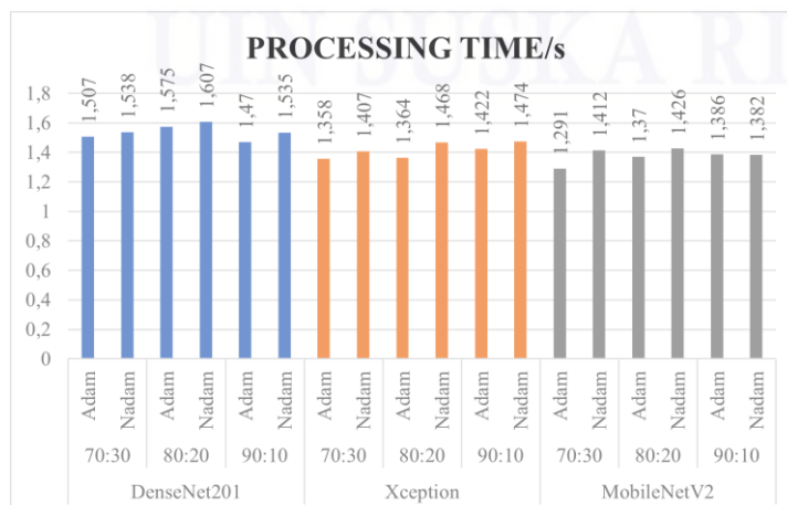
Gambar 8. Waktu Pelatihan Arsitektur
