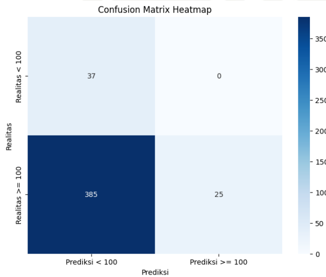
Gambar 5 Hasil dari Teknik split validation 70:30
