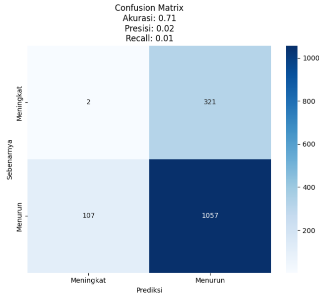
Gambar 4 Hasil dari 10-Fold Cross Validation
