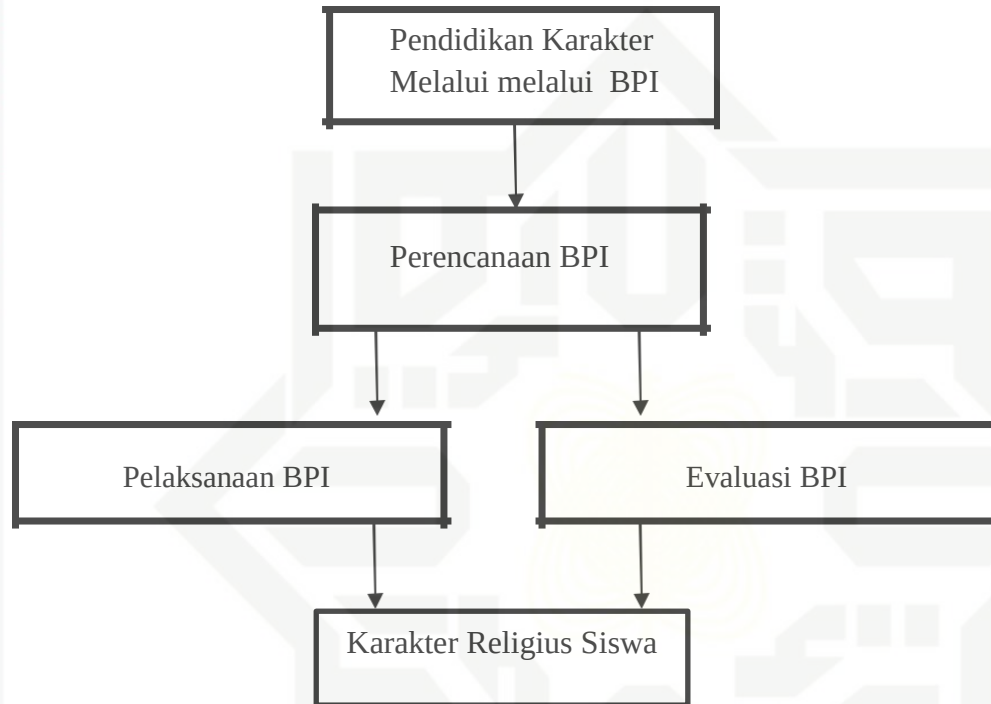
Gambar 2. 1 Kerangka Teori
