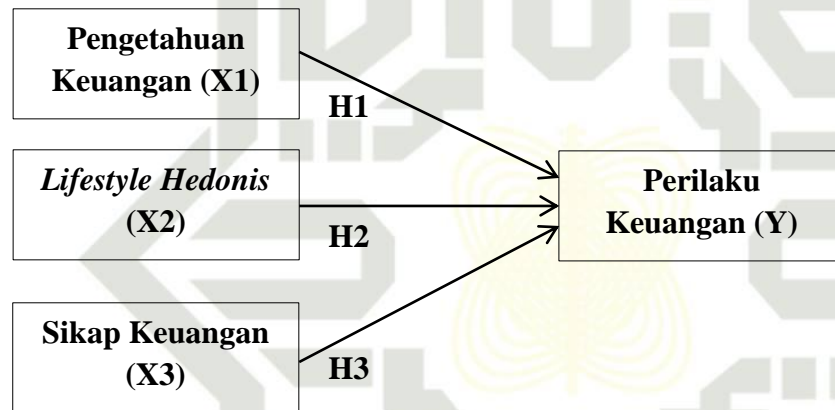
Gambar 2.2 Kerangka Pemikiran
