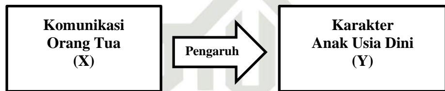
Gambar 2.2 Kerangka Pemikiran
