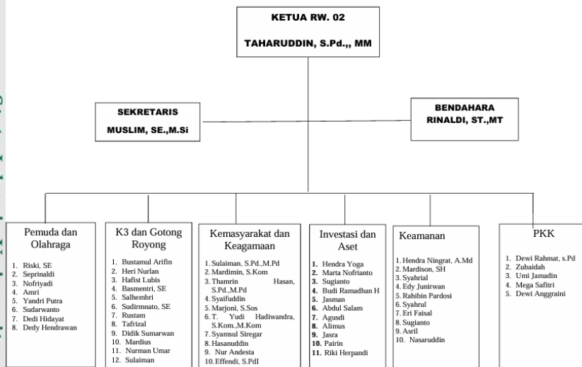
Gambar 4.1 Struktur Organisasi
