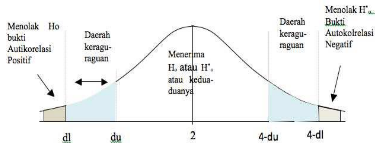
Gambar 3.1 Daerah dalam Uji Durbin Watson
