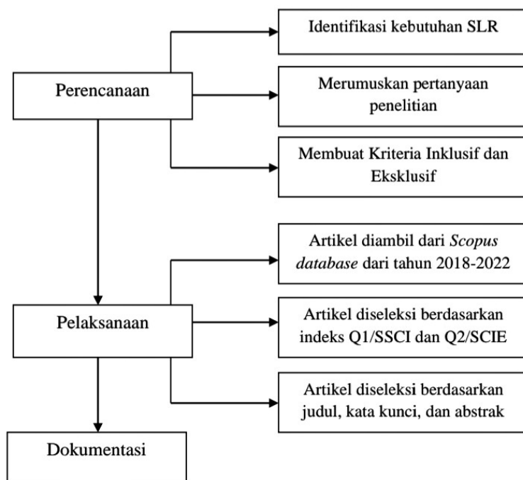
Gambar 3.1. Metodologi Penelitian
