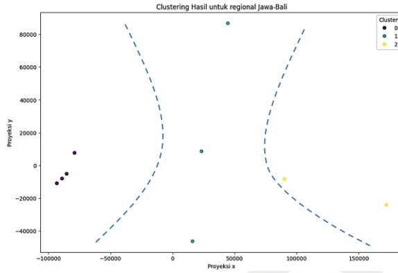
Gambar 3. scatter plot Klasterisasi Regional Jawa-Bali.
