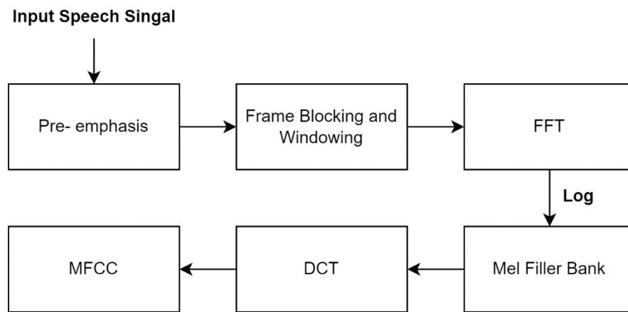
Gambar 2. 2 Alur Ekstraksi Fitur MFCC
