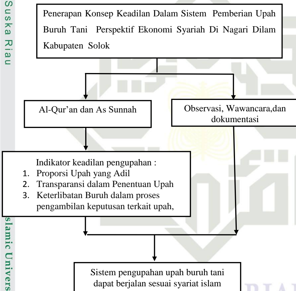
Gambar II.I Kerangka Berpikir
