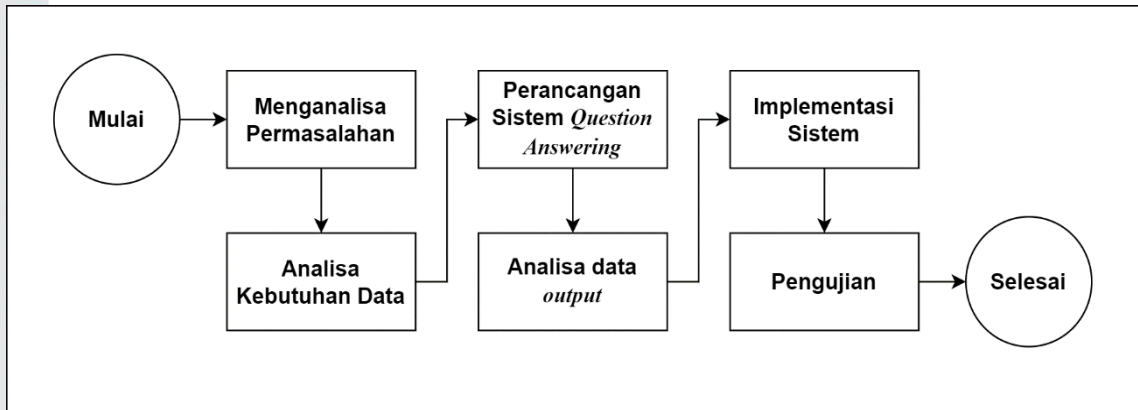
Gambar 1. Metodologi Penelitian
