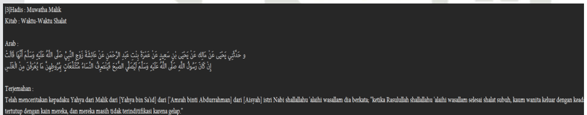
Gambar 2. Data Awal
