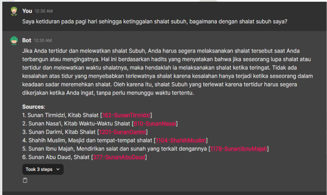
Gambar 5. Jawaban Sistem
