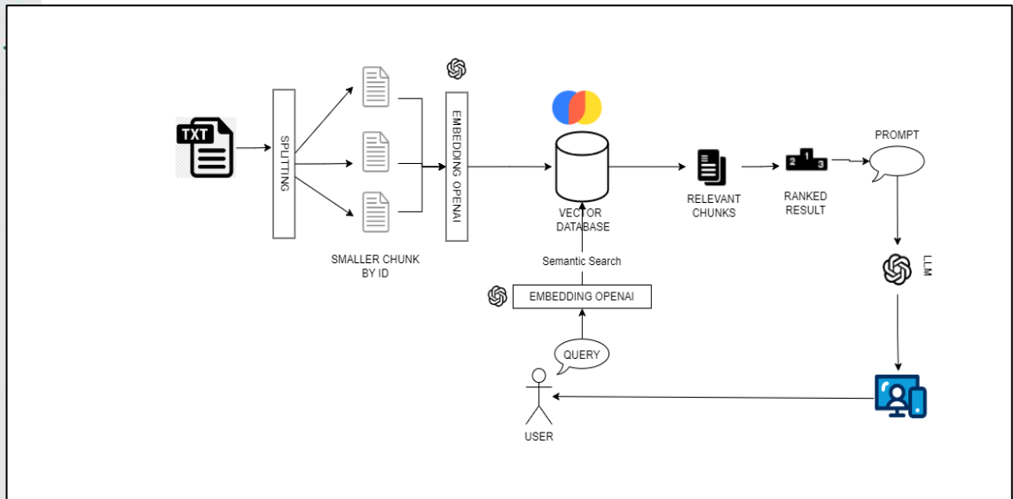
Gambar 3. Alur Sistem
