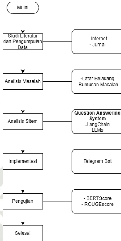
Gambar 1. Tahapan Penelitian
