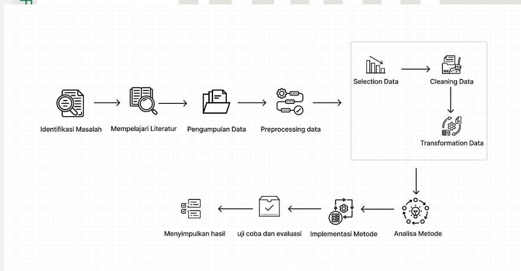
Gambar 3. 1 Metodologi Penelitian
