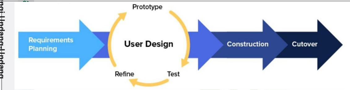
Gambar 2 Metode RAD
