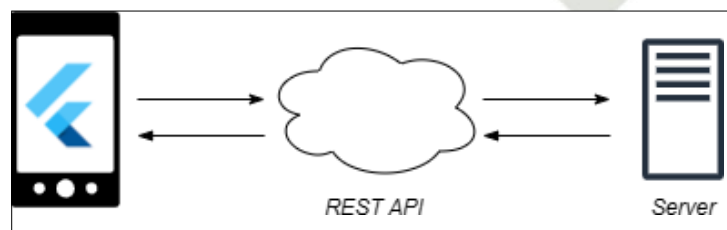
Gambar 3 Skema Aplikasi
