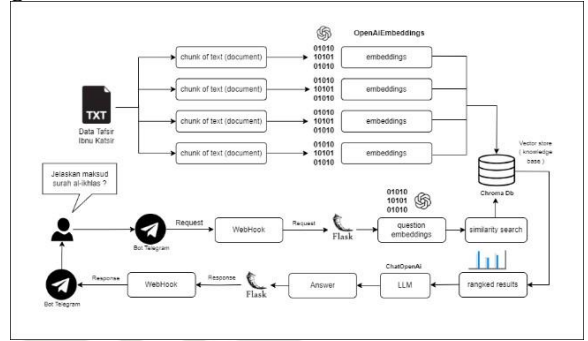
Gambar 4. Alur Kerja Sistem
