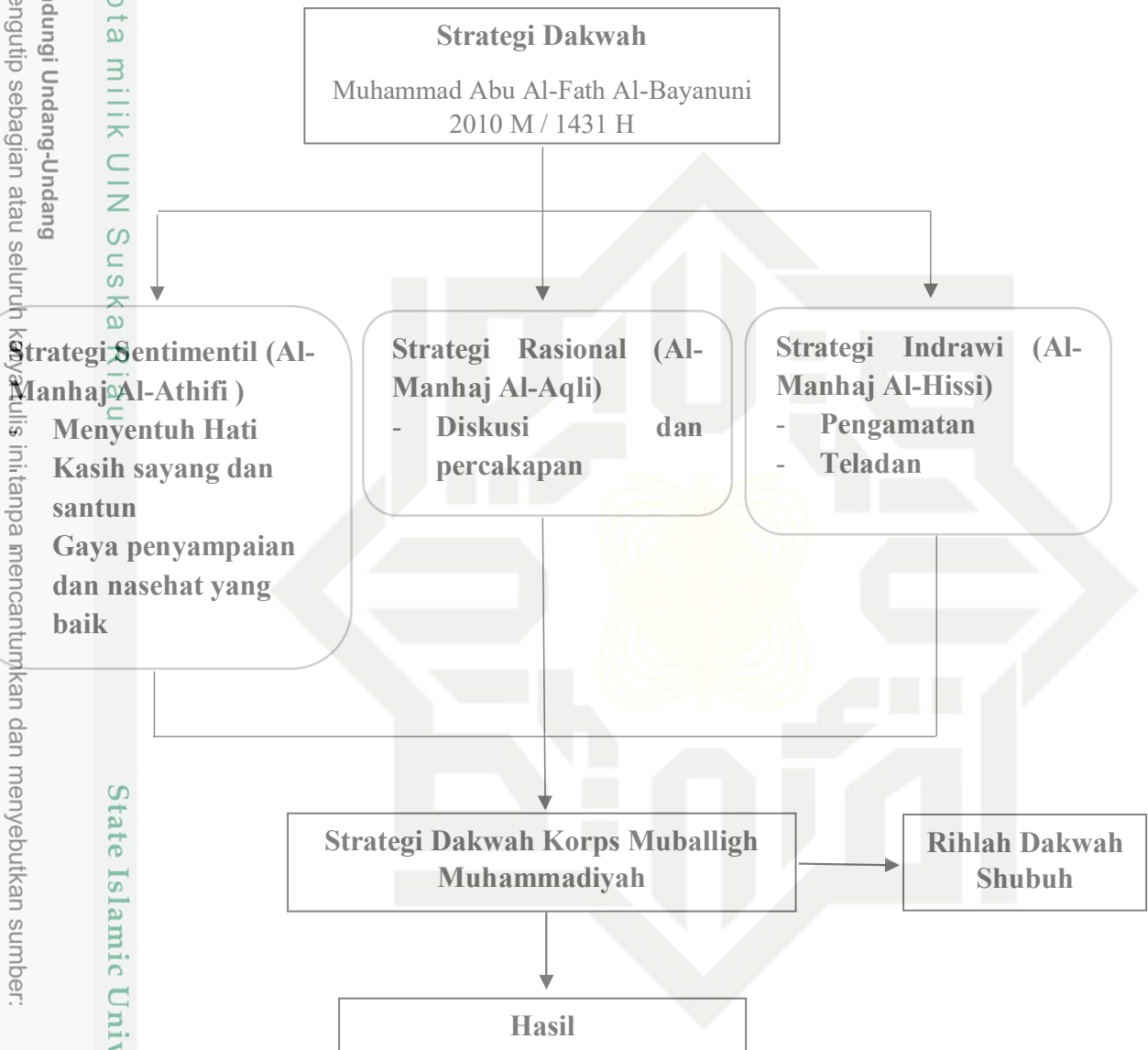
Bagan 2.1
