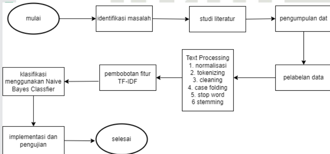
Gambar 3.1 Metodologi Penelitian
