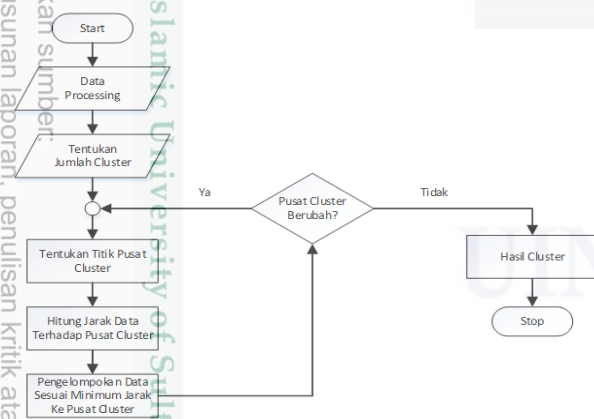
Gambar 2. Tahap Algoritma K-Means
