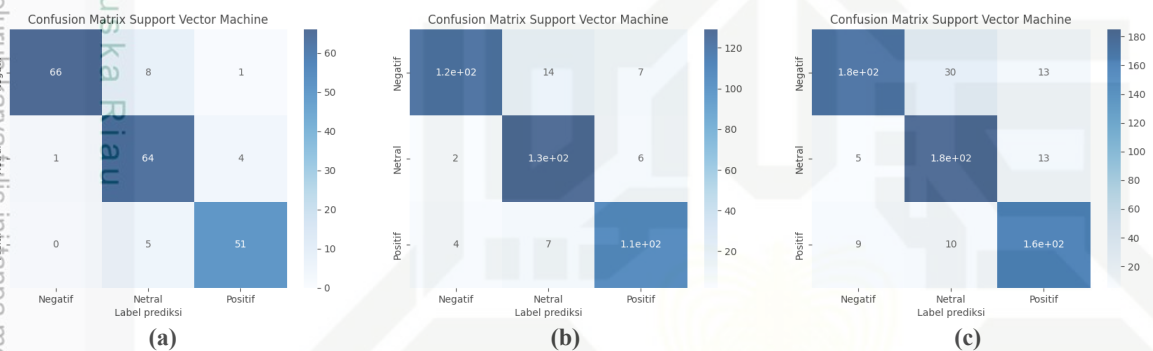
Gambar 6 Confusion Matrix model Support Vector Machine dengan pembagian data latih dan uji (a) 90 :10 (b) 80:20 dan (c) 70:30
