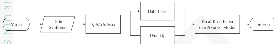
Gambar 4. Flowchart klasifikasi
