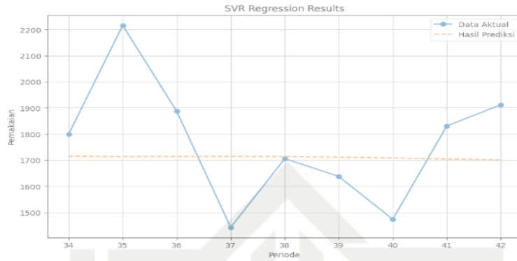
Grafik 7. Hasil Prediksi Terhadap Bulan Obat Paracetamol 500 mg - SVR
