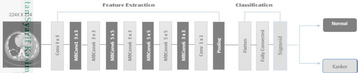
Gambar 5. Arsitektur EfficientNet-B0
