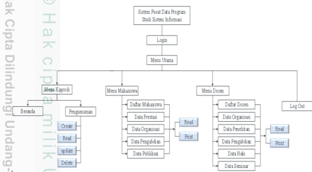
Gambar 4. Rancangan menu kaprodi
