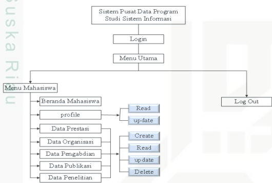
Gambar 6. Rancangan menu mahasiswa
