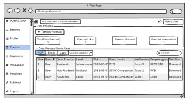
Gambar 18. Halaman data prestasi
