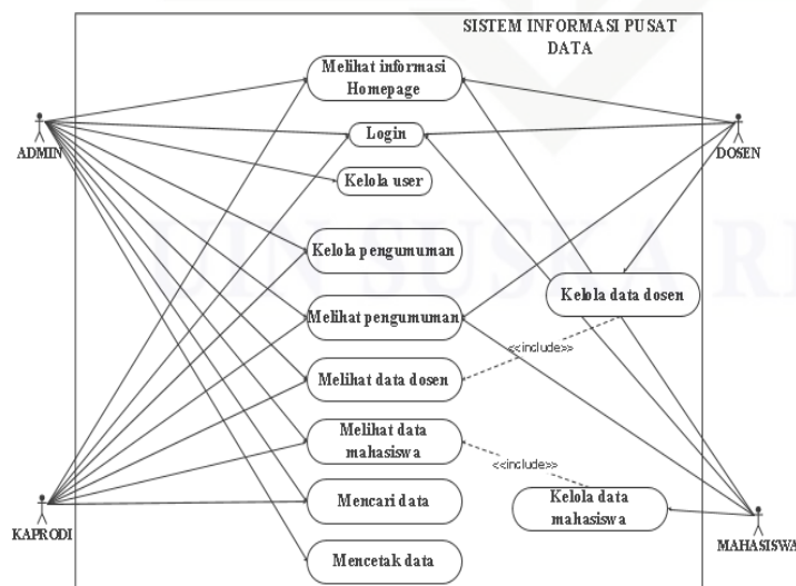
Gambar 2. Use case diagram sistem informasi pusat data
