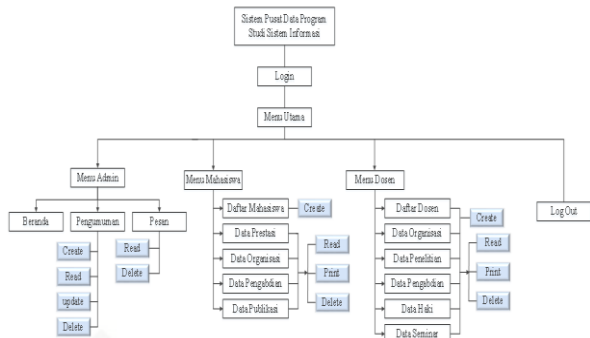
Gambar 5. Rancangan menu admin
