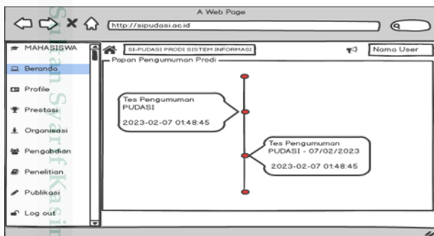
Gambar 17. Halaman beranda mahasiswa
