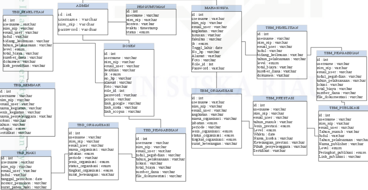
Gambar 8. Rancangan database sistem pusat data
