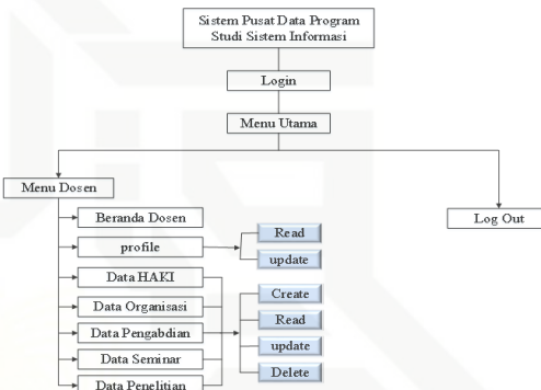
Gambar 7. Rancangan menu dosen
