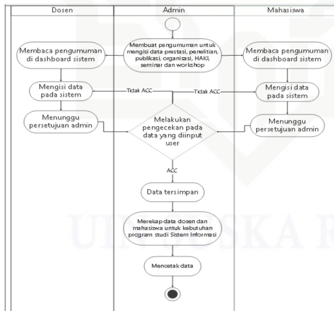
Gambar 3. Diagram aktivitas sistem informasi pusat data
