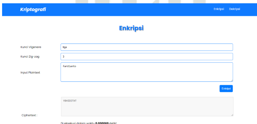
Gambar 6. Proses Enkripsi
