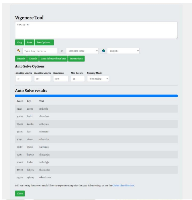
Gambar 8. Pengujian Ciphertext
