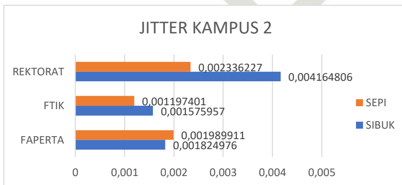
Gambar 11. Grafik Nilai Jitter Kampus 2
