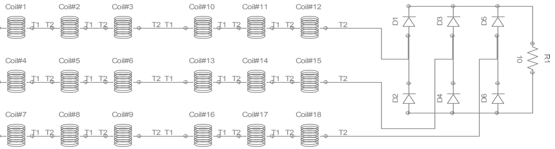
Gambar 6. Circuit / Rangkaian Pembebanan PMSG 18S16P
