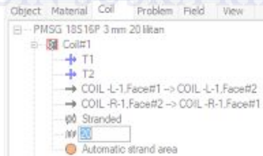
Gambar 5. Mengatur Coil 20 Lilitan
