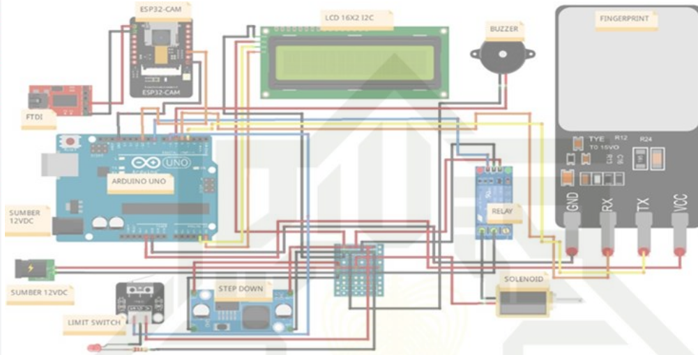
Gambar 2. Skema Interkoneksi pada Komponen
