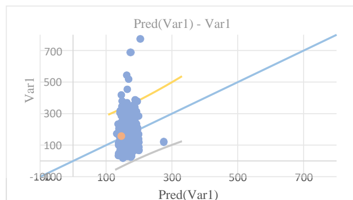
Gambar 5. Pred (Var1)
