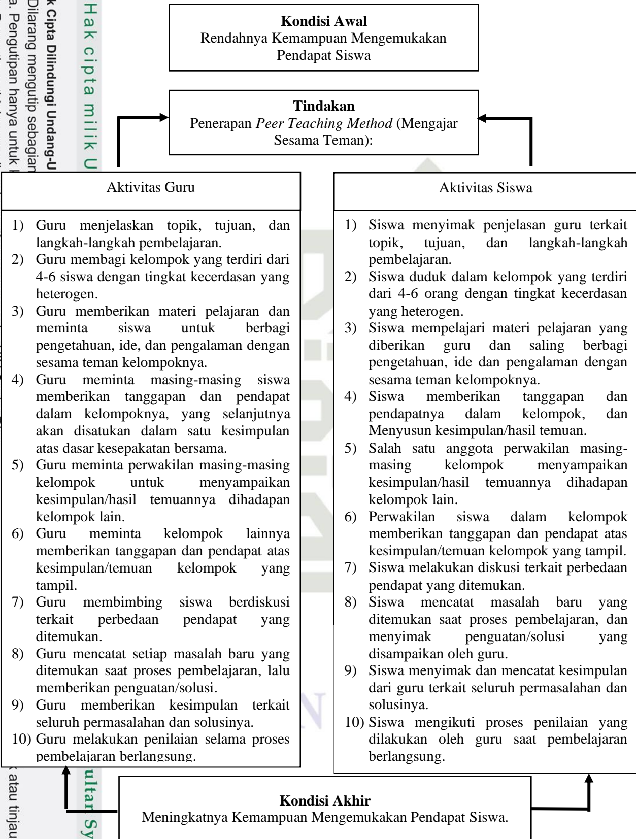
Gambar II.1 Kerangka Berpikir
