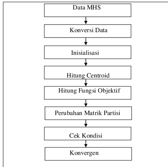
Gambar 4.1 Tahapan Algoritma Fuzzy C-Means
