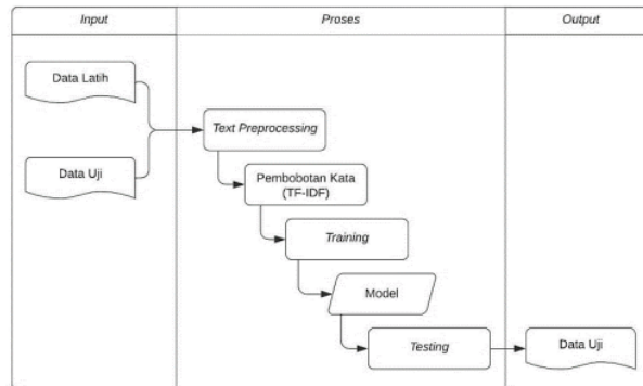
Gambar 3. Alur Tahapan Klasifikasi K-Nearest Neighbor
