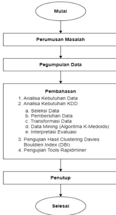
Gambar 1. Metodologi Penelitian
