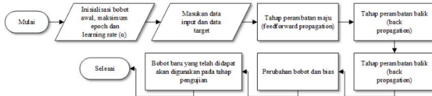
Gambar 2. Langkah-Langkah Pelatihan Metode Backpropagation
