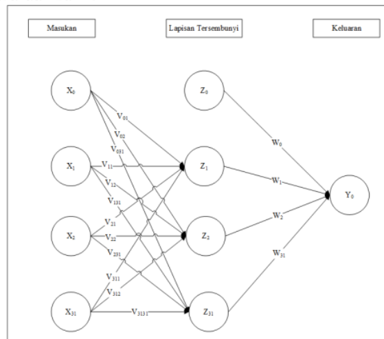
Gambar 4. Arsitektur jaringan backpropagation
