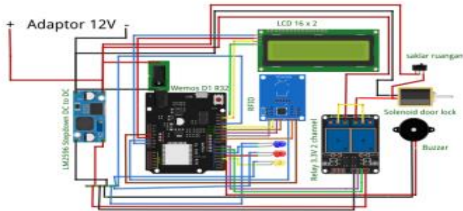
Gambar 2. Diagram pengkabelan
