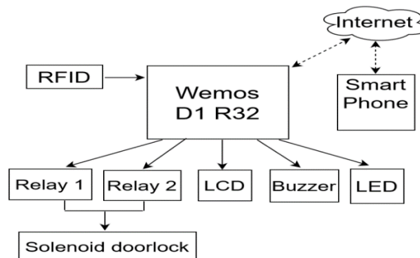
Gambar 1. Blok diagram perangkat keras
