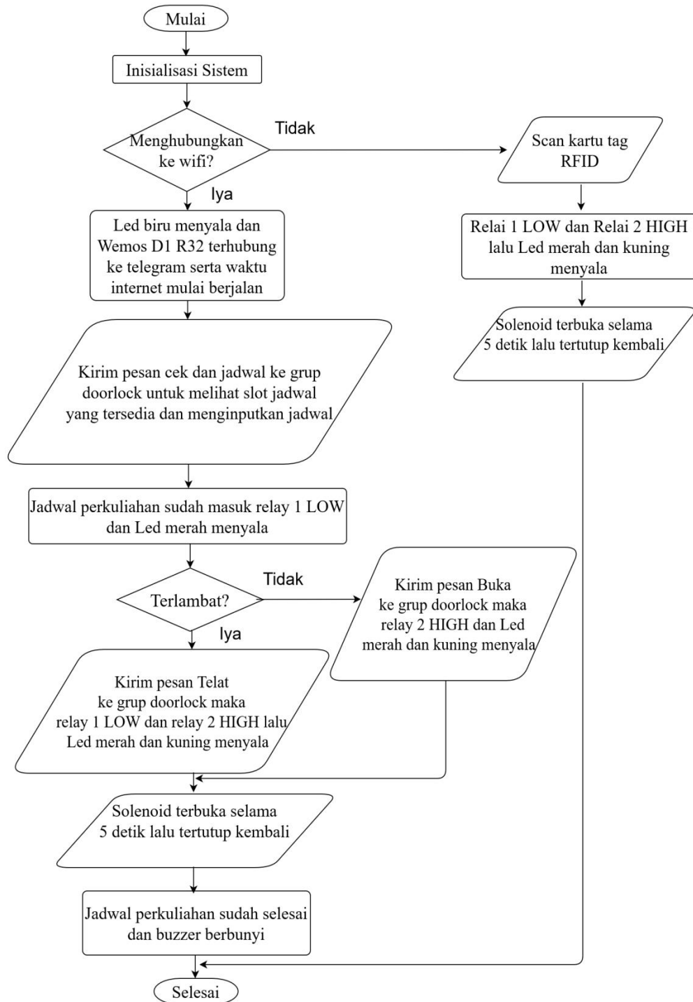
Gambar 4. Flowchart perangkat lunak
