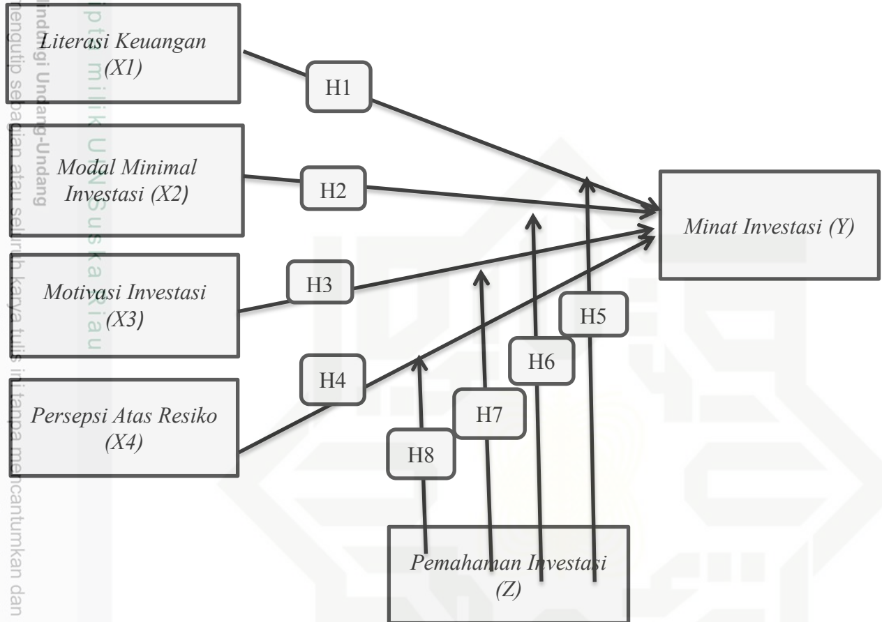
Gambar 1 Kerangka Penelitian
