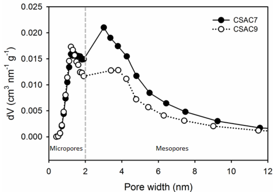
Gambar 4.4 Profil ukuran pori CSAC7 dan CSAC9
