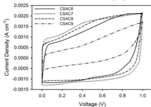
41 42 43 44 45 46 47 48 49 50 51 52 53 54 55 56 57 58 59 60 Figure 5. CV curve of CSAC6, CSAC7, CSAC8, and CSAC9
