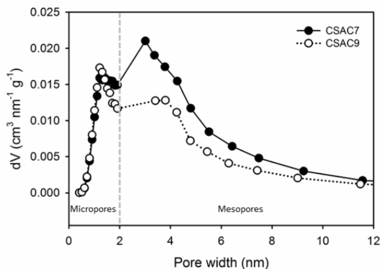
Gambar 4.4 Profil ukuran pori CSAC7 dan CSAC9
