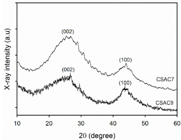
Gambar 4.1 Pola XRD dari Sampel CSAC7 dan CSAC9
