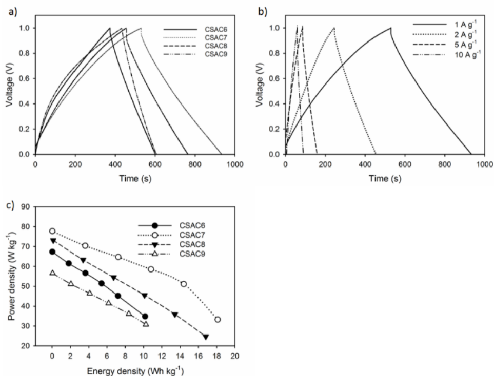
Gambar 4.7 (a) Kurva GCD CSAC6, CSAC7, CSAC8, dan CSAC9, (b) Kurva GCD pada kerapatan arus CSAC7 yang berbeda, dan (c) Plot Ragone dari CSAC6, CSAC7, CSAC8, dan CSAC9 dalam 1 M elektrolit H 2 SO 4
