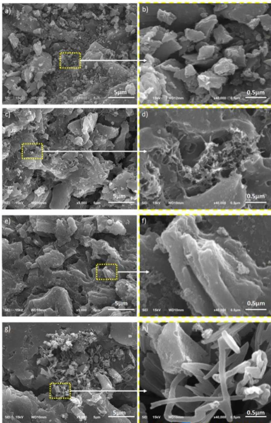
24 Gambar 4.2 Makrograf SEM CSAC6 dalam pembesaran (a) 5.000x, (b) 40.000x, CSAC7 dalam pembesaran (c) 5.000x, (d) 40.000x, CSAC8 dalam pembesaran (e) 5.000x, (f) 40.000x, CSAC9 dalam pembesaran (g) 5.000x, (h) 40.000x
