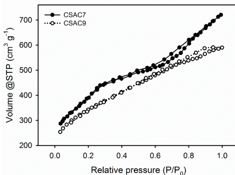
Gambar 4.3 Isoterm Adsorpsi-Desorpsi Nitrogen CSAC7 dan CSAC9
