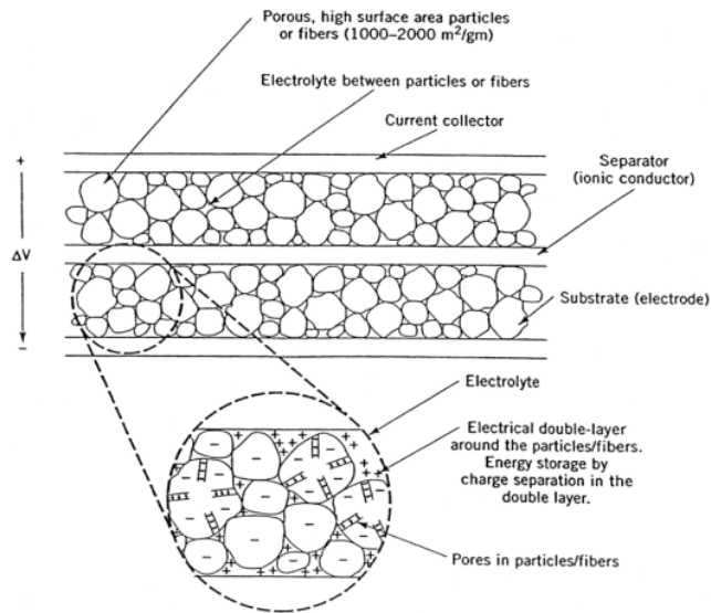
Gambar 2.2. Struktur superkapasitor
