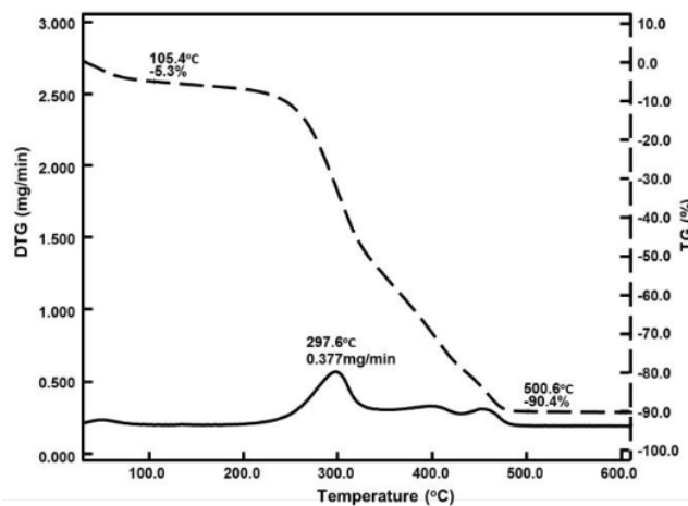
Gambar 4.1. kurva TG/DTG untuk serbuk pra-karbon rumput gajah
