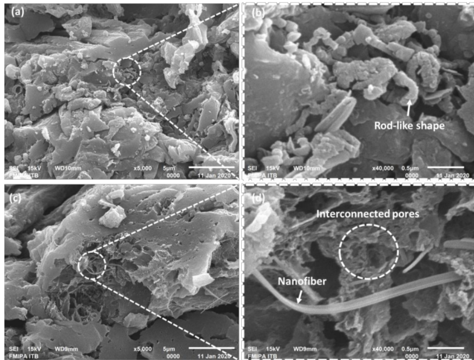
Gambar 4.4. SEM mikrograf untuk (a) MG0.3, (b) perbesaran dari MG0.3, (c) MG0.5, (d) perbesaran dari MG0.5
