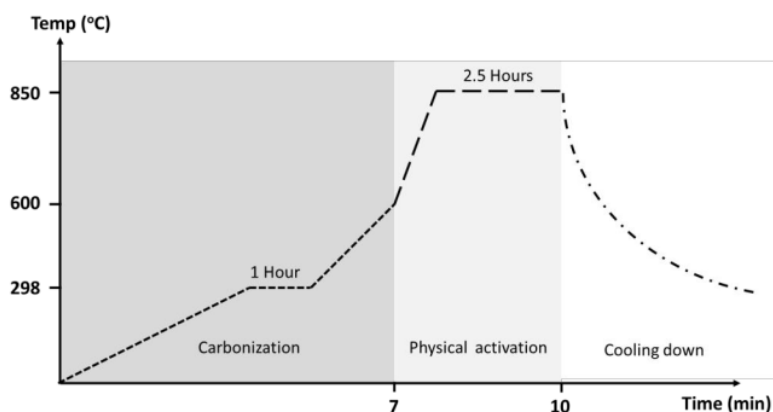
Gambar 4.2. Profil proses pirolisis satu tahap
