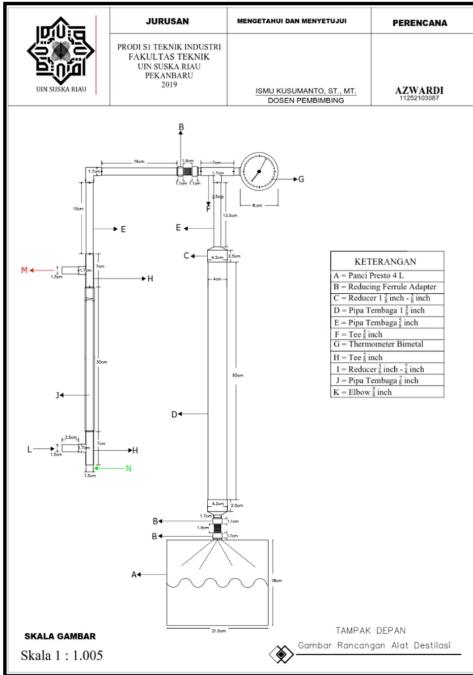
Gambar 2. Sketsa Rancangan Alat Destilasi.
