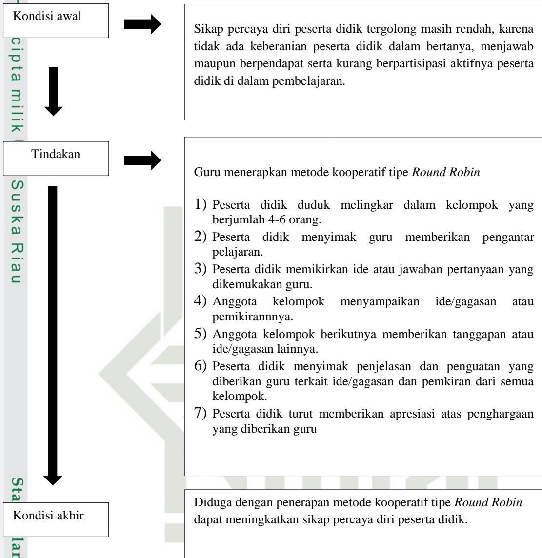
Gambar II.1 Kerangka Berfikir
