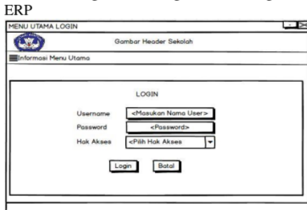
Gambar D.3 Perancangan Menu Login Sistem Integrasi ERP
