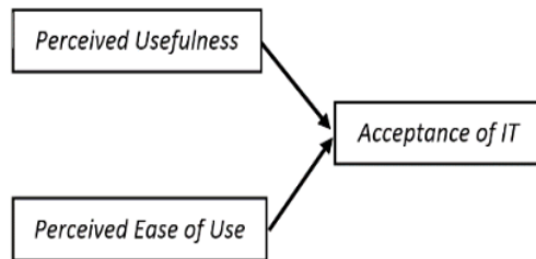
Gambar 3. Kerangka Penelitian
