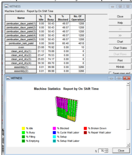
Gambar 9. Laporan kinerja mesin layout awal
