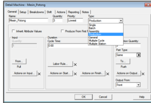
Gambar 4. Detail machine untuk mesin potong papan kayu
