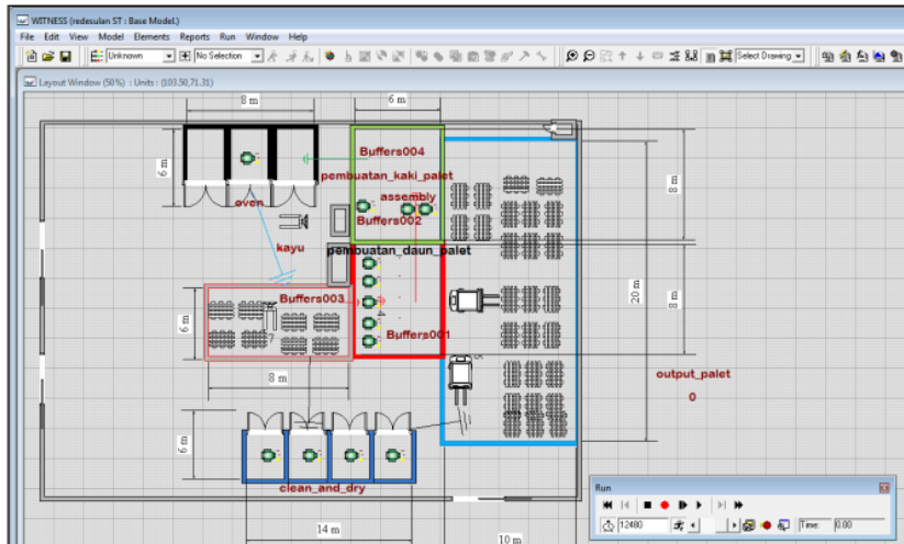
Gambar 6. Susunan Model keseluruhan Layout Usulan
