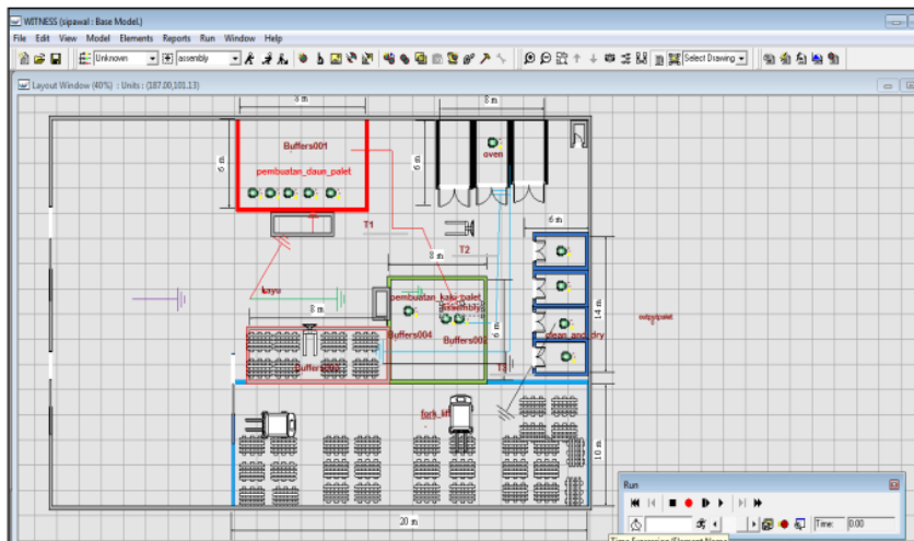
Gambar 5. Susunan model keseluruhan layout awal
