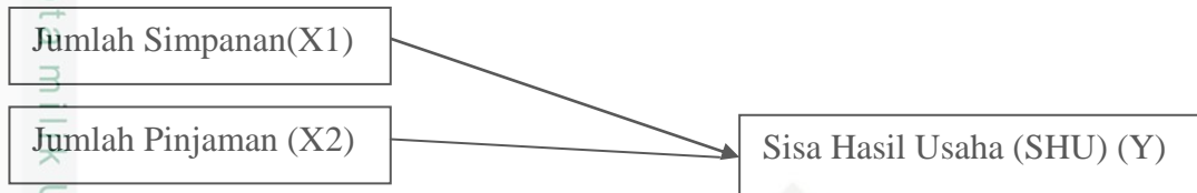
Gambar II.1 Kerangka Pikir
