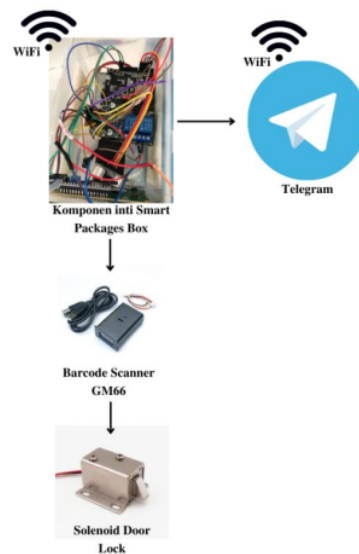
Gambar 3. Rancangan Perangkat Keras
