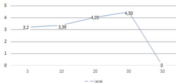
Gambar 10. Grafik Pengukuran Jarak GM 66
