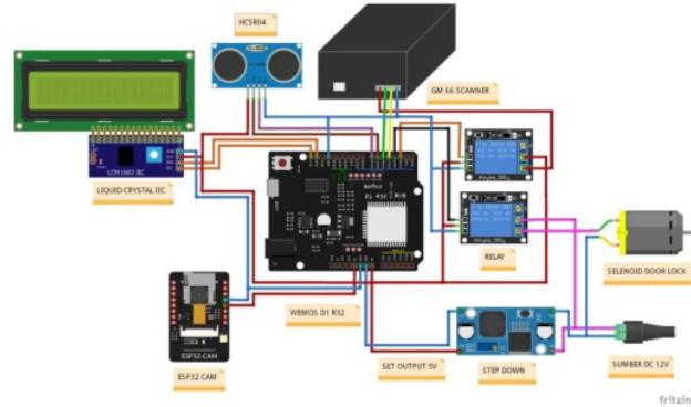
Gambar 4. Rangkaian Skematik Smart Packages Box
