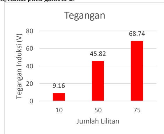
Gambar 2. Perbandingan Tegangan Setiap Variasi Lilitan
