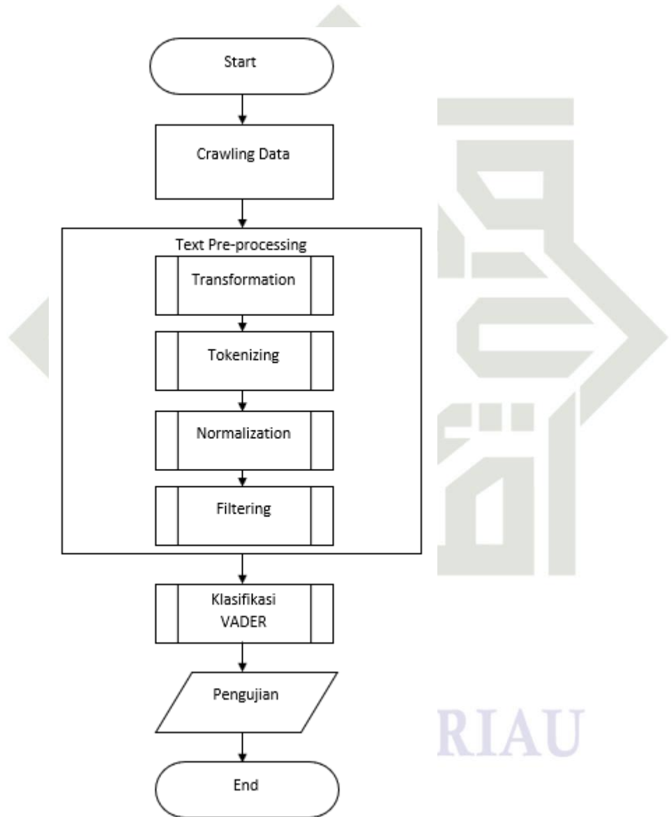
Gambar 3.1 Tahapan Metodologi Penelitian
